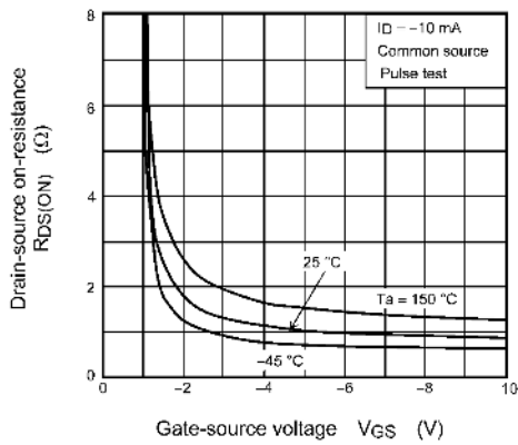
Fig. 7.3 R_{DS(ON)} - V_{GS}
