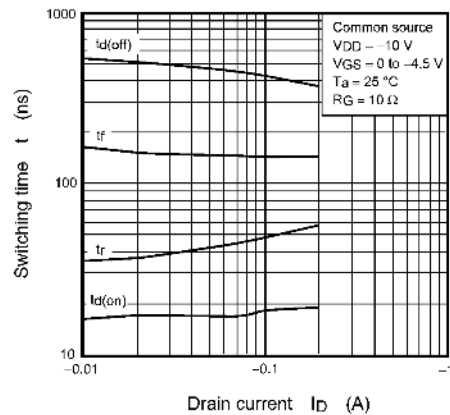
Fig. 7.10 t - I_D
