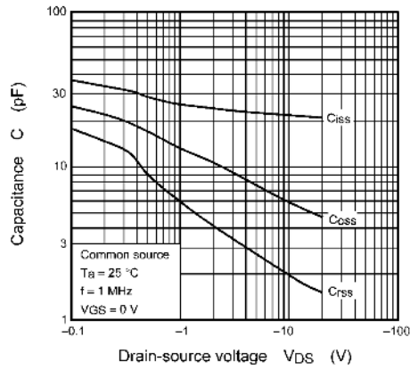
Fig. 7.9 C - V_{DS}
