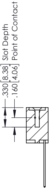
SECTION A-A
