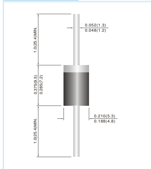
DO-201AD Unit : inch(mm)
