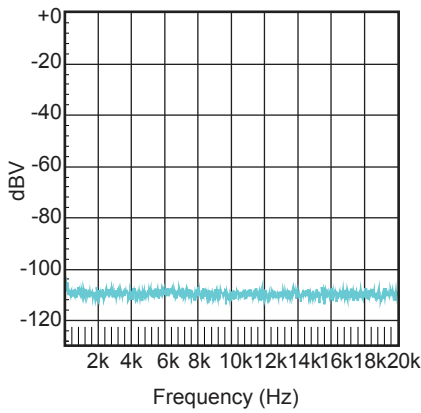
FFT Noise Floor Test (12V, 4Ω+33μH)
