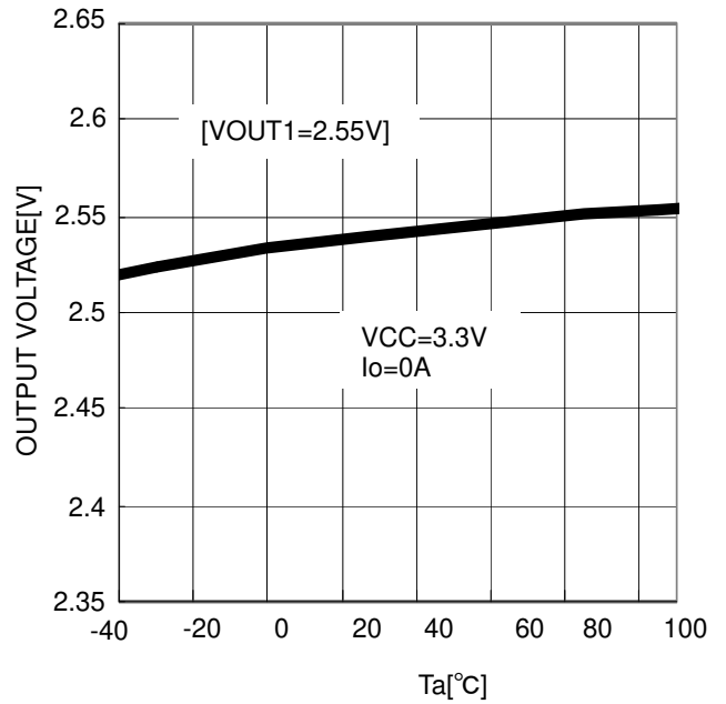
Figure.7 Ta-VOUT1
