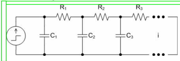
Fig. 14. Cauer Thermal Network
