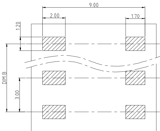
P.C.B. LAYOUT
