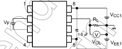
Fig. 12.1.4 VOL Test Circuit
