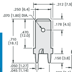
.250 (6.4) TAB
