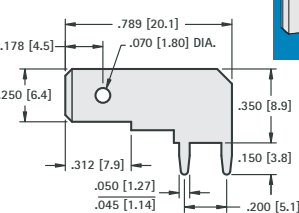
.250 (6.4) TAB
