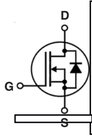
TO-263 AA (IXTA)
