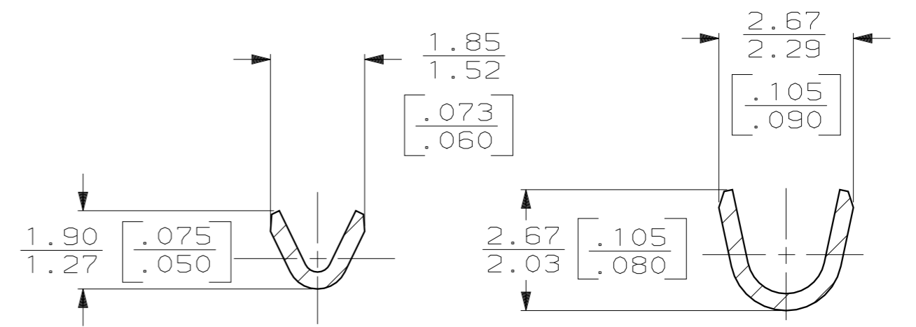
SECTION A-A SCALE 10:1
