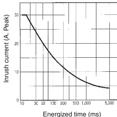
G3TA-OA202SZ/OA202SL-US
