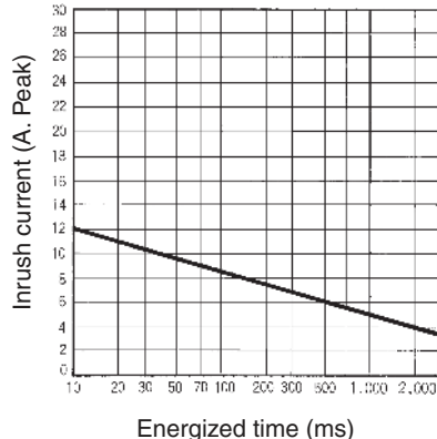
G3TA-ODX02S-US
