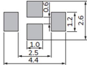
NFM31PC/31KC
