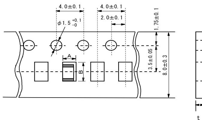
(3)GRT18/21/31/32(Paper Tape)
