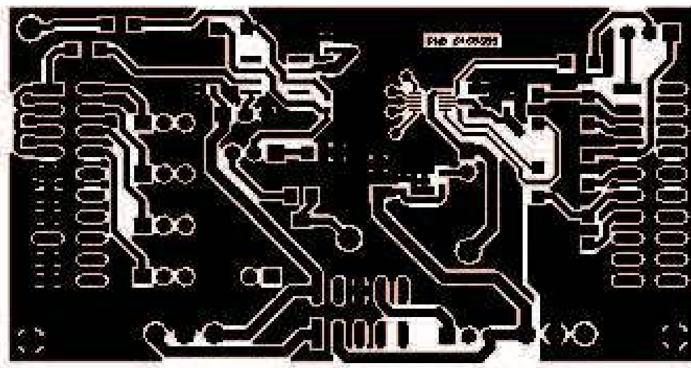
DAC7554 REV A LAYER 1 TOP SIGNAL LAYER
