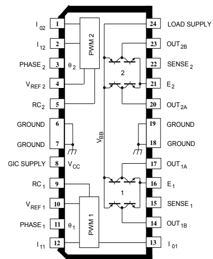
Dwg. PP-047
