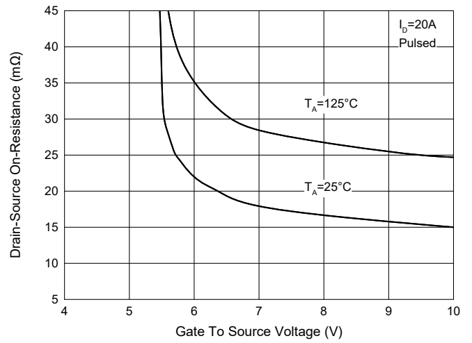
Fig. 2 - R_{DS(ON)} - V_{GS}
