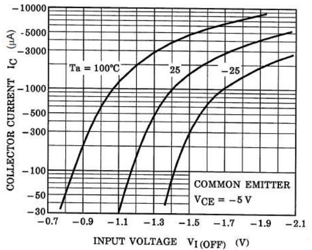
Fig. 10.10 RN2304 I_C - V_{I(OFF)}
