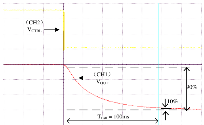
V_{CTRL} : 0.25V ~ 5V V_{OUT} : 1250V ~ 25000V
