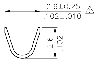
SEC: A-A
