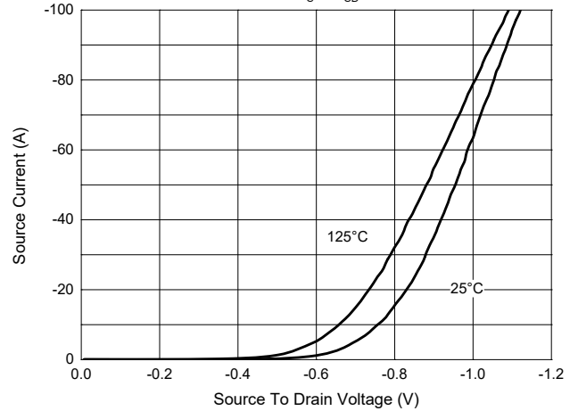
Fig. 4 - I_s - V_{SD}
