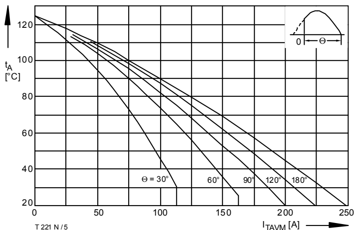
Bild / Fig. 5 Höchstzulässige Kühlmitteltemperatur / Max. allowable cooling medium temperature t_A = f(I_{TAVM}) Verstärkte Luftkühlung / forced air cooling Kühlkörper / Heatsink: K0.55-FB54-A, V_L = 50 \text{ l/s} Parameter: Stromflußwinkel / Current conduction angle \theta
