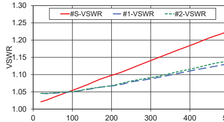
ZFSC-2-1-S+ VSWR
