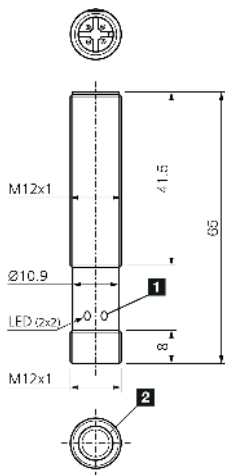
1) LED 2 x 2 2) Schallaustritt Ultraschallwandler BK: schwarz BN: braun BU: blau WH: weiß
