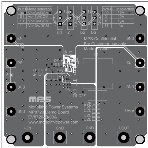
Figure 1—Top Layer
