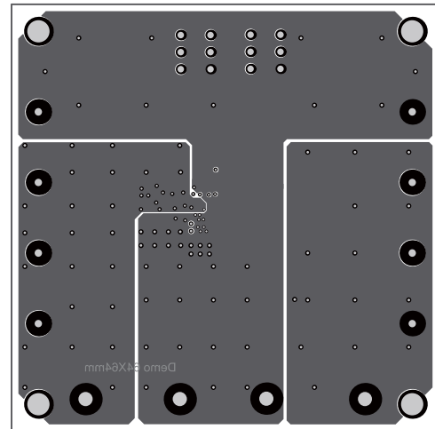
Figure 4—Bottom Layer
