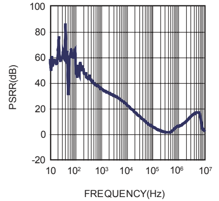
PSRR
