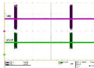
TPS25963x 1KV EFT Response
