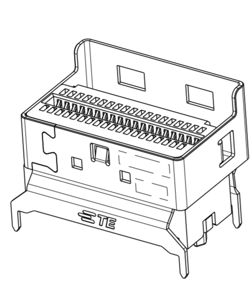
W/O DUST CAP SCALE 4:1
