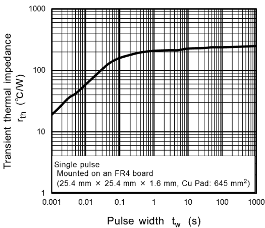
Fig. 8.10 r_{th} - t_w
