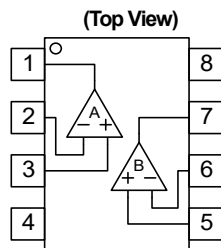
NJM2903CG / NJM2903CAG NJM2903CM / NJM2903CAM NJM2903CRB1 / NJM2903CARB1 NJM2903CV / NJM2903CAV
