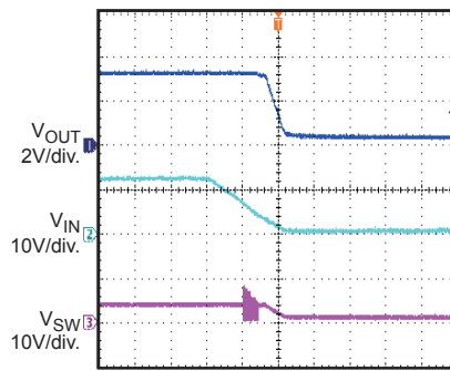
VIN Shutdown
