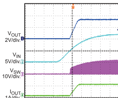
VIN Startup
