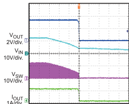
VIN Shutdown
