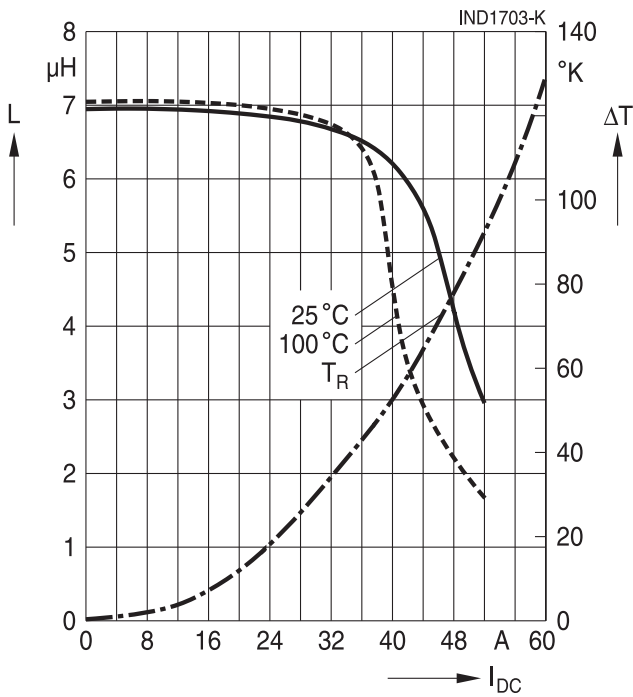
B82559B6682A027
