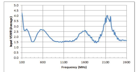
VSWR
