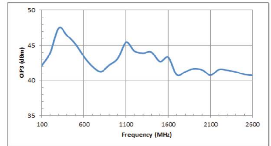
OIP3
