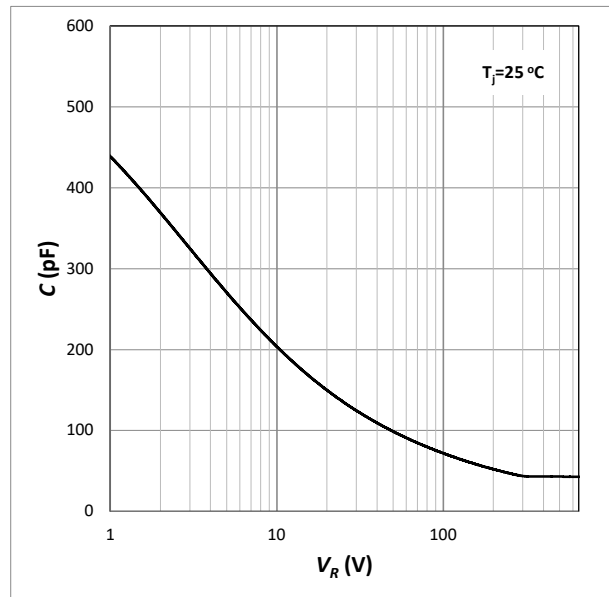
Fig. 6 Capacitance
