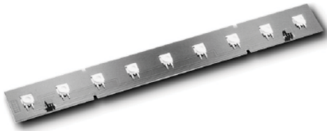
ADJD-xM30 (9 LEDs)
