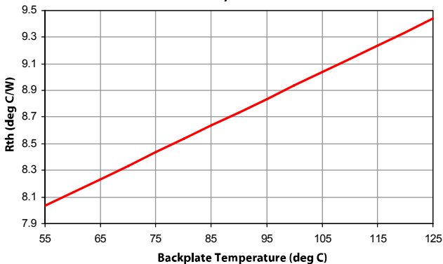
XP1027-BD Vd=6.0 V, Id1=200 mA Id2=500 mA, Id3=1100 mA
