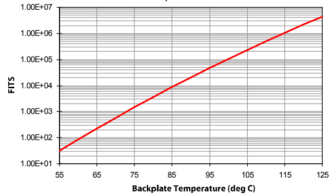
XP1027-BD Vd=6.0 V, Id1=200 mA Id2=500 mA, Id3=1100 mA
