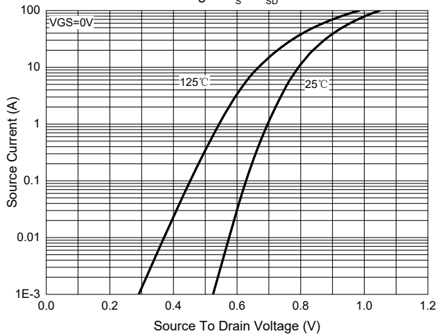
Fig.9 - I_S - V_{SD}
