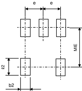
SSOP5
