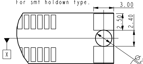
DETAIL E SCALE 3.000
