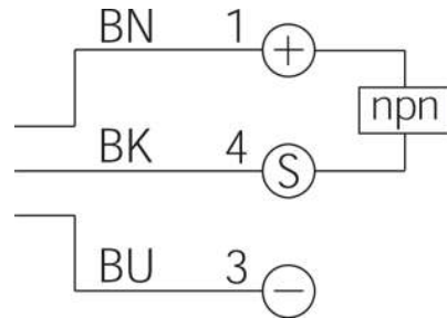
1) LED 4 x 90° (gelb) 2) Schlüsselweite 17 mm BK: schwarz BN: braun BU: blau
