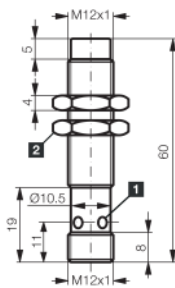
1) LED 4 x 90° (gelb) 2) Schlüsselweite 17 mm BK: schwarz BN: braun BU: blau
