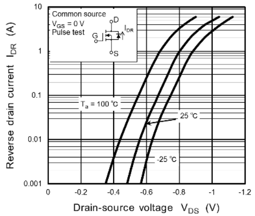
Fig. 7.10 I_{DR} - V_{DS}
