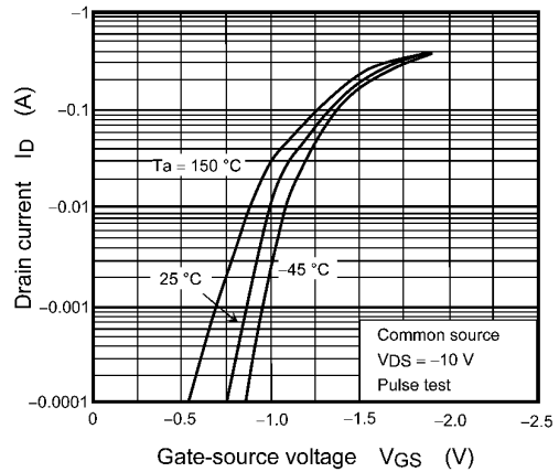
Fig. 9.2 I_D - V_{GS}
