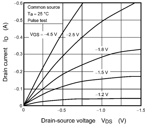
Fig. 9.1 I_D - V_{DS}
