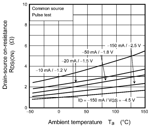
Fig. 9.5 R_{DS(ON)} - T_a
