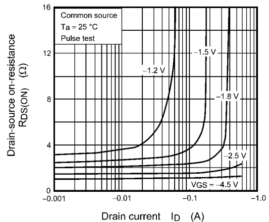
Fig. 9.6 R_{DS(ON)} - I_D
