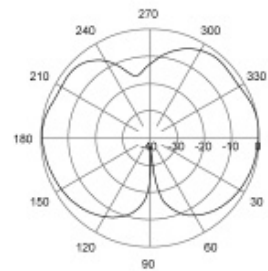
E-Plane | 420 MHz
