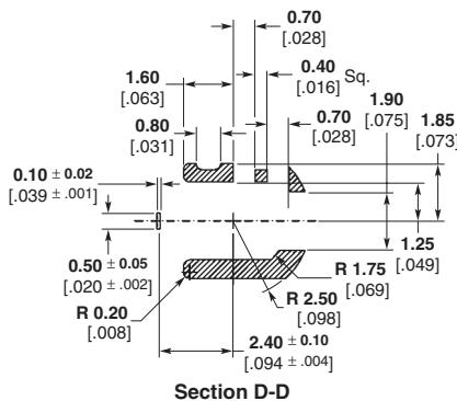
Section D-D
