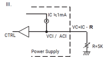
External Resistor (KΩ)
