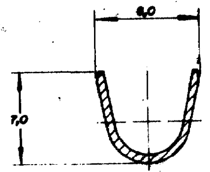
SECCÃO-C-C
