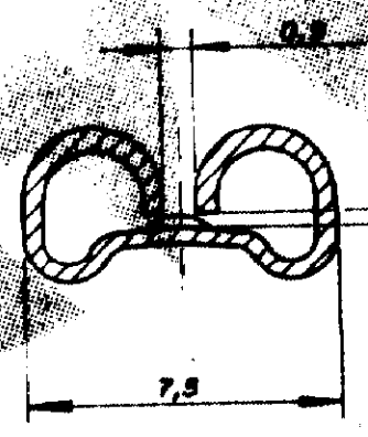
SECCÃO-A-A
