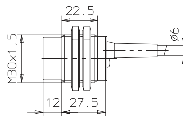
E2EL-X15M□ 2M
