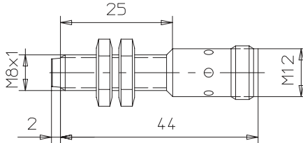
E2EL-X2M□-M1
