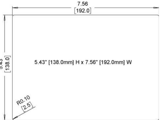
Cutout Dimensions
