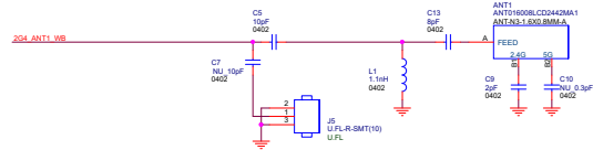
WL_BG/BT ANT1
