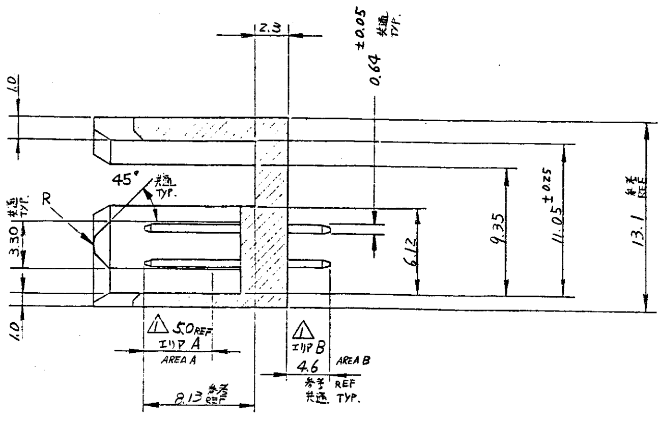
断面 X-X SECTION X-X
