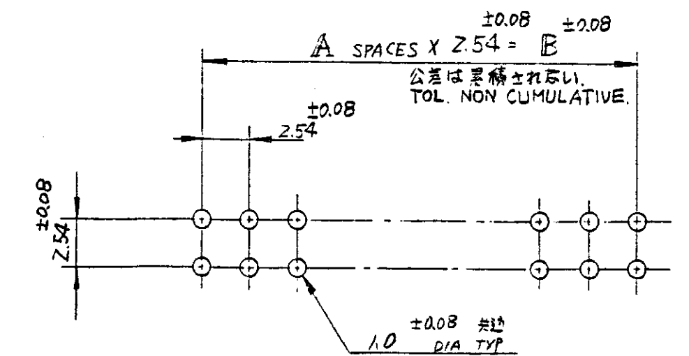
プリント基板推奨穴位置 RECOMMENDED HOLE LAYOUT
